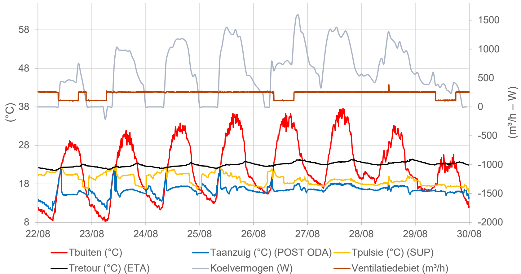
Koelvermogen tov ventilatiedebiet 22-30 augustus
